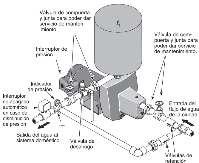
Figura 7: Modelo SNCPI5
