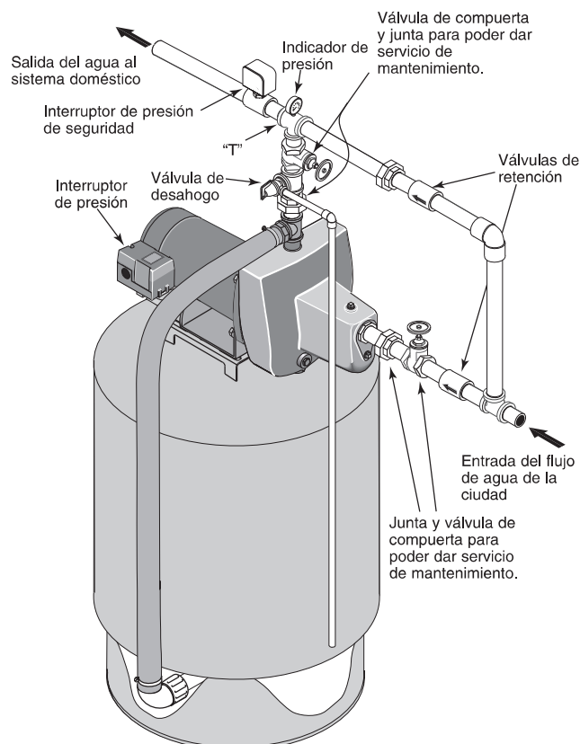
Figura 6: Modelo SNCP42
