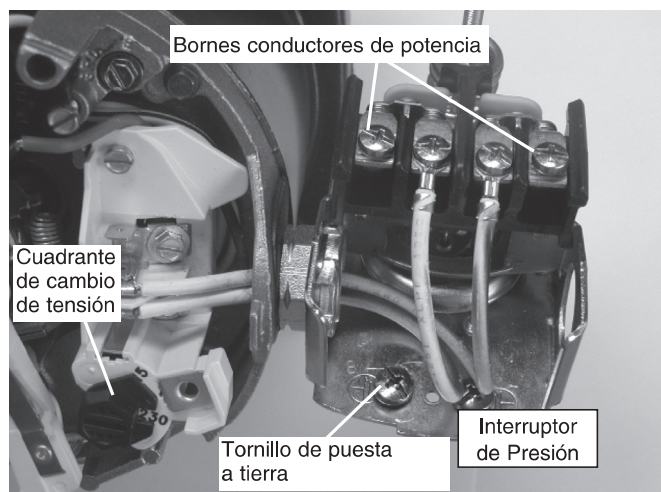
Figura 9: Cuadrante de regulación de tensión
