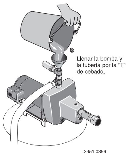
Figura 9: Llenado de la Bomba
