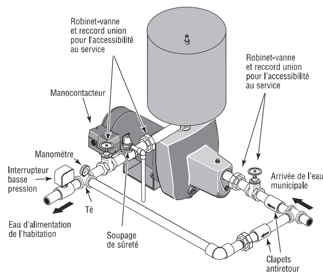
Figure 7: Modèle SNCP15
