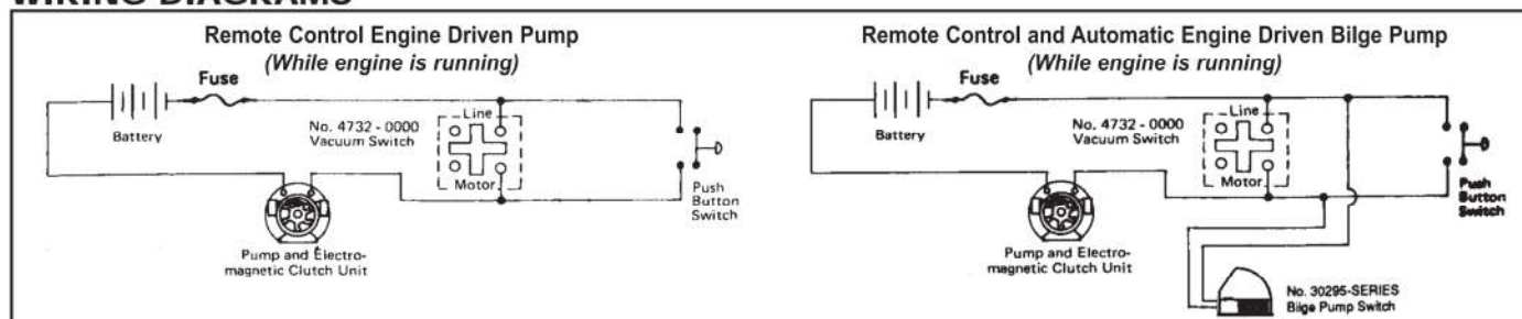
WIRING DIAGRAMS
